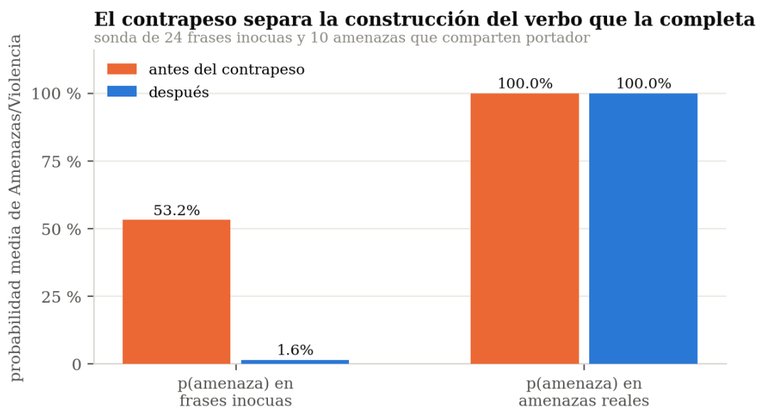
Figura 10 Efecto del contrapeso sobre la sonda de construcción
