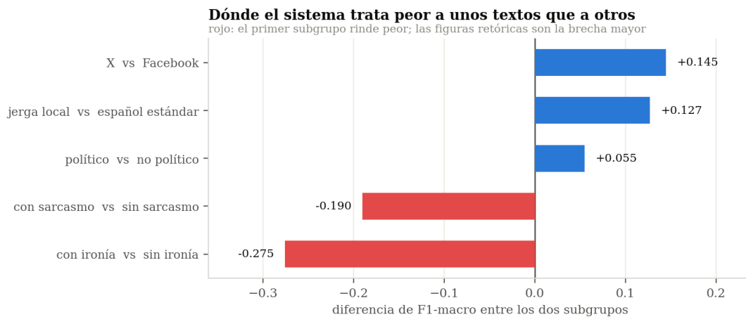
Figura 11 Brechas de desempeño entre subgrupos del conjunto de prueba
