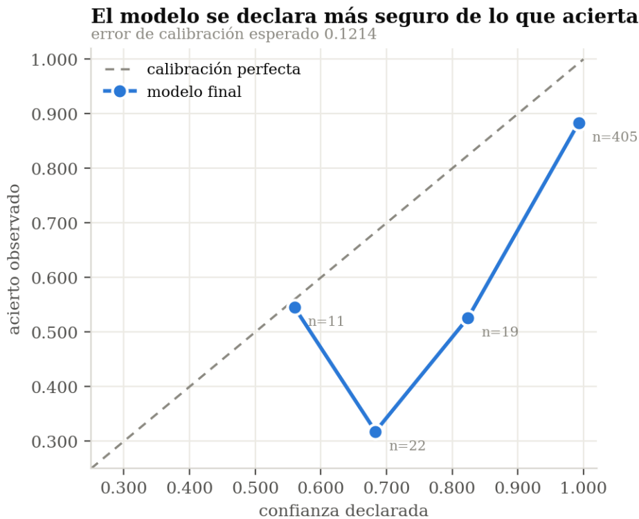
Figura 12 Confianza declarada frente a acierto observado
